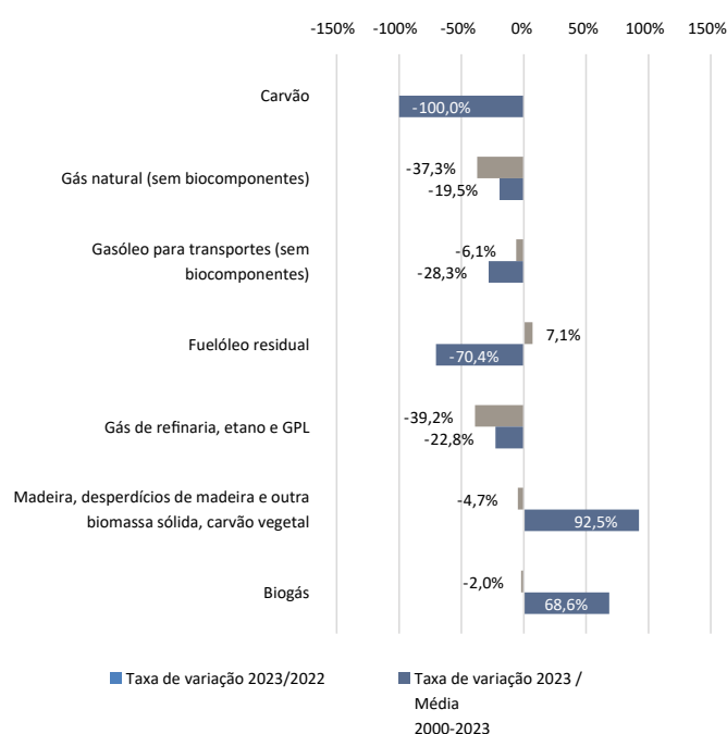
Recursos energéticos naturais utilizados na transformação em energia elétrica
